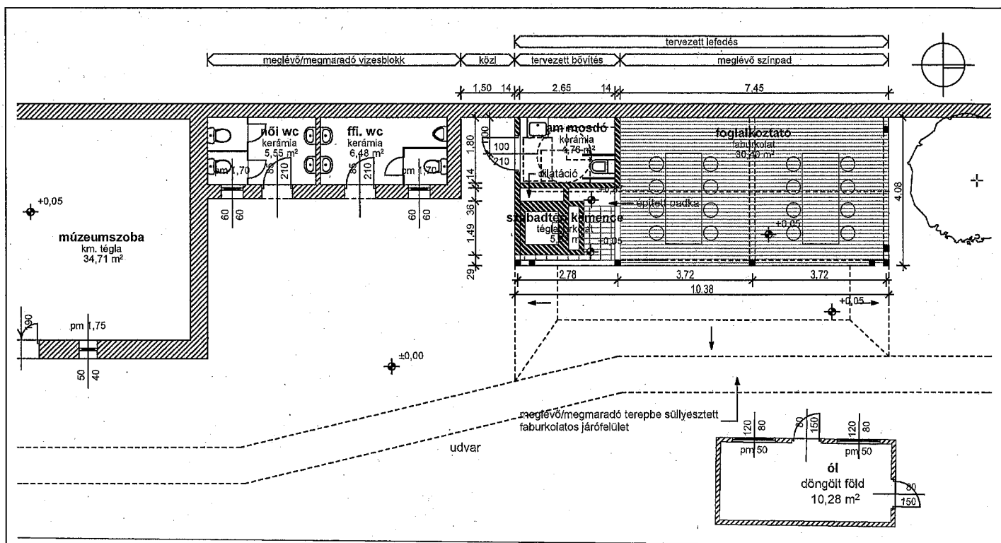
alaprész
