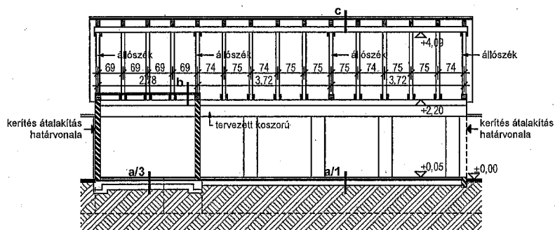
hosszmetszet
