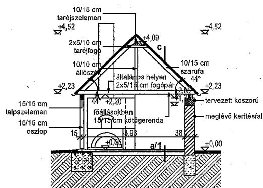
keresztmetszet foglalkoztatón keresztül
