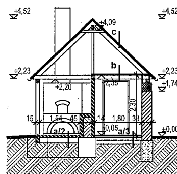
keresztmetszet vizesblokkon keresztül
