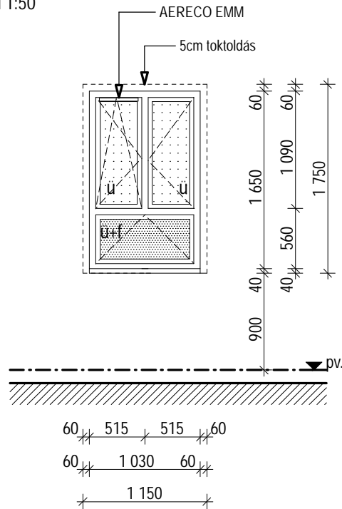
NÉZET M 1:50
