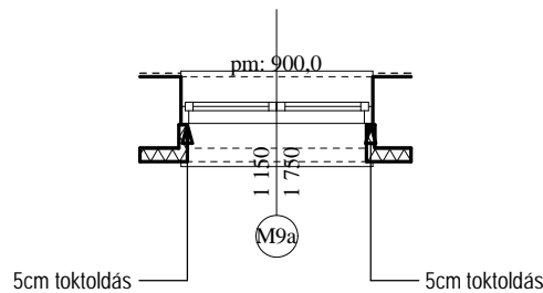
ALAPRAJZ M 1:50
