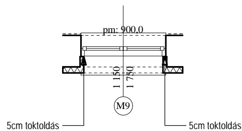
ALAPRAJZ M 1:50
