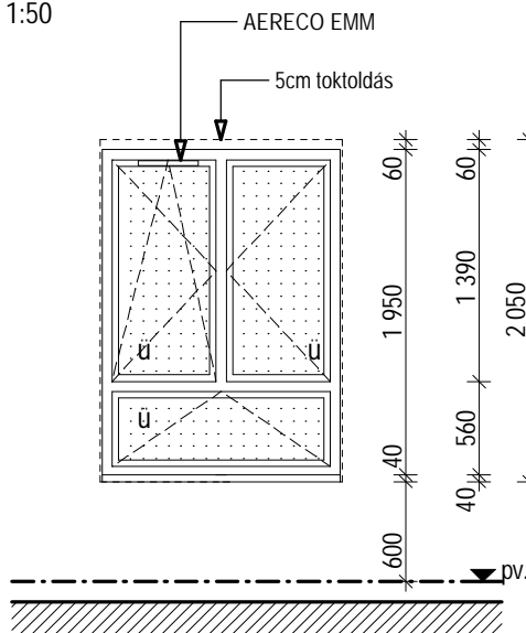
NÉZET M 1:50
