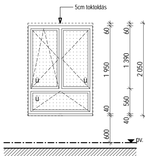
NÉZET M 1:50
