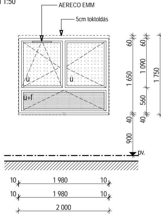
NÉZET M 1:50
