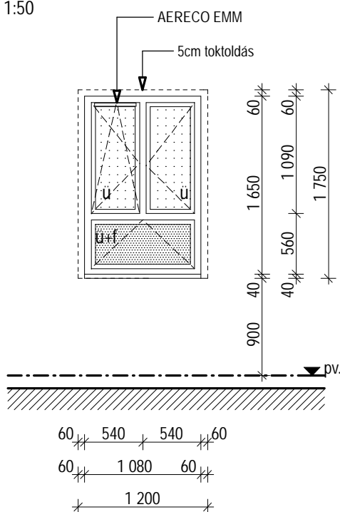
NÉZET M 1:50
