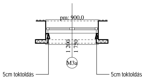
ALAPRAJZ M 1:50
