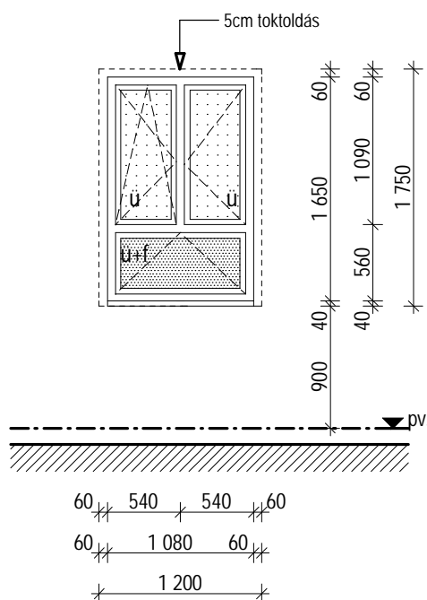
NÉZET M 1:50
