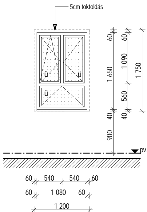
NÉZET M 1:50
