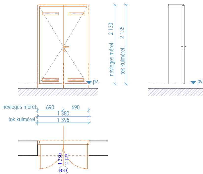
METSZET M 1:50
