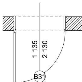
ALAPRAJZ M 1:50
