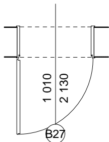
ALAPRAJZ M 1:50
